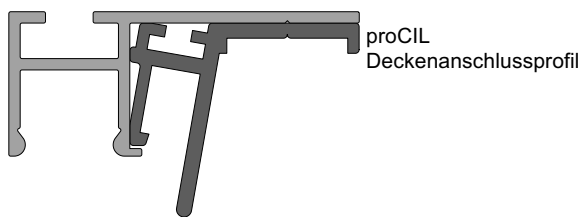
Lichtkanal proCIL Wandanschlussprofil
